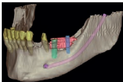
Computergestützte Planungssoftware.
